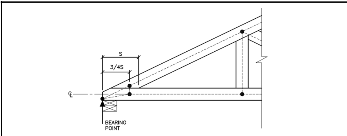
Figure 4.1.2.1.B Girder Heel
